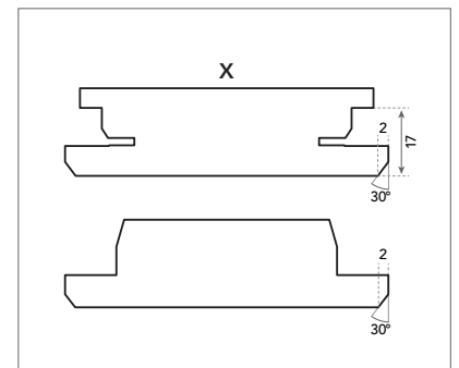
El sistema de perfilera oculta con canto simétrico X garantiza un montaje rápido en ambas direcciones.
